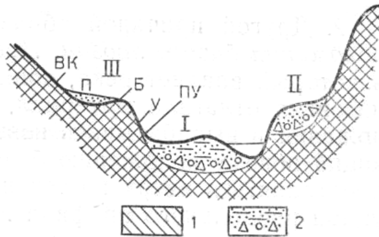
1- коренные породы; 2 – аллювиальные отложения
