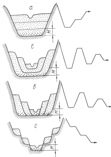
Рис. 21. Долины аккумулятивные (а, б, в) и смешанная (г)
