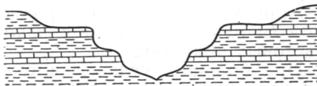
Рис. 20. Скульптурные террасы (профиль)
