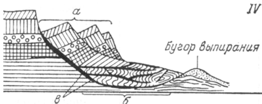
а - деляпсивная часть; б - детрузивная часть; в – зона брекчирования
