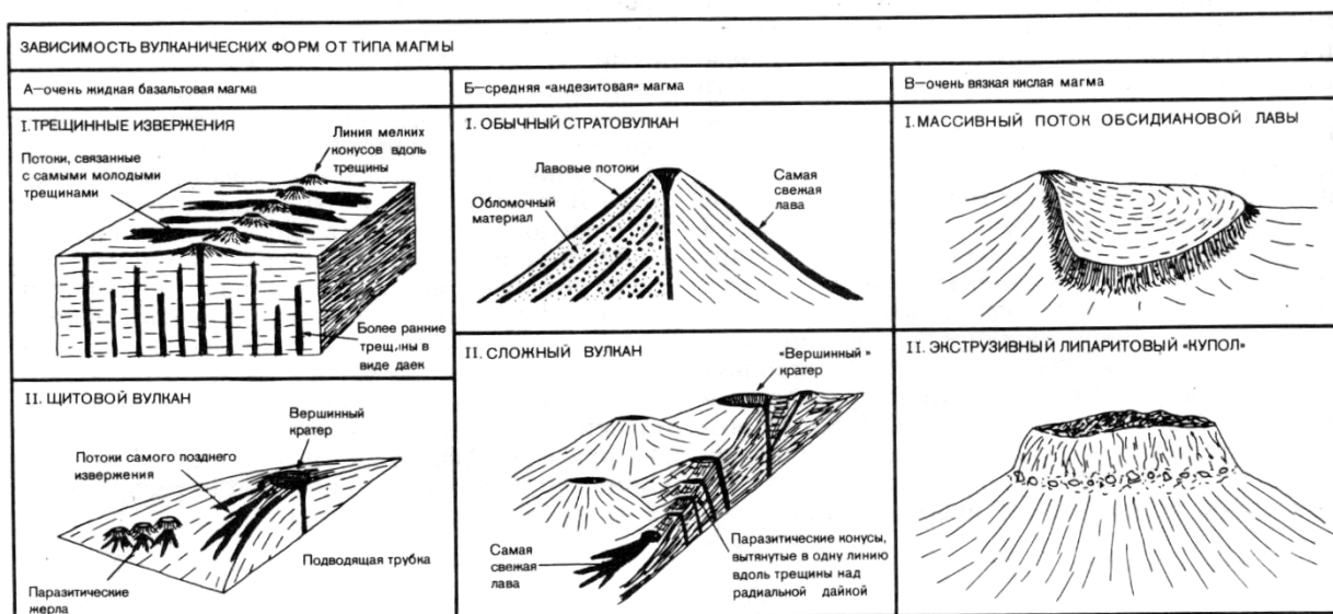
Рис. 3. Рельеф, созданный вулканами
