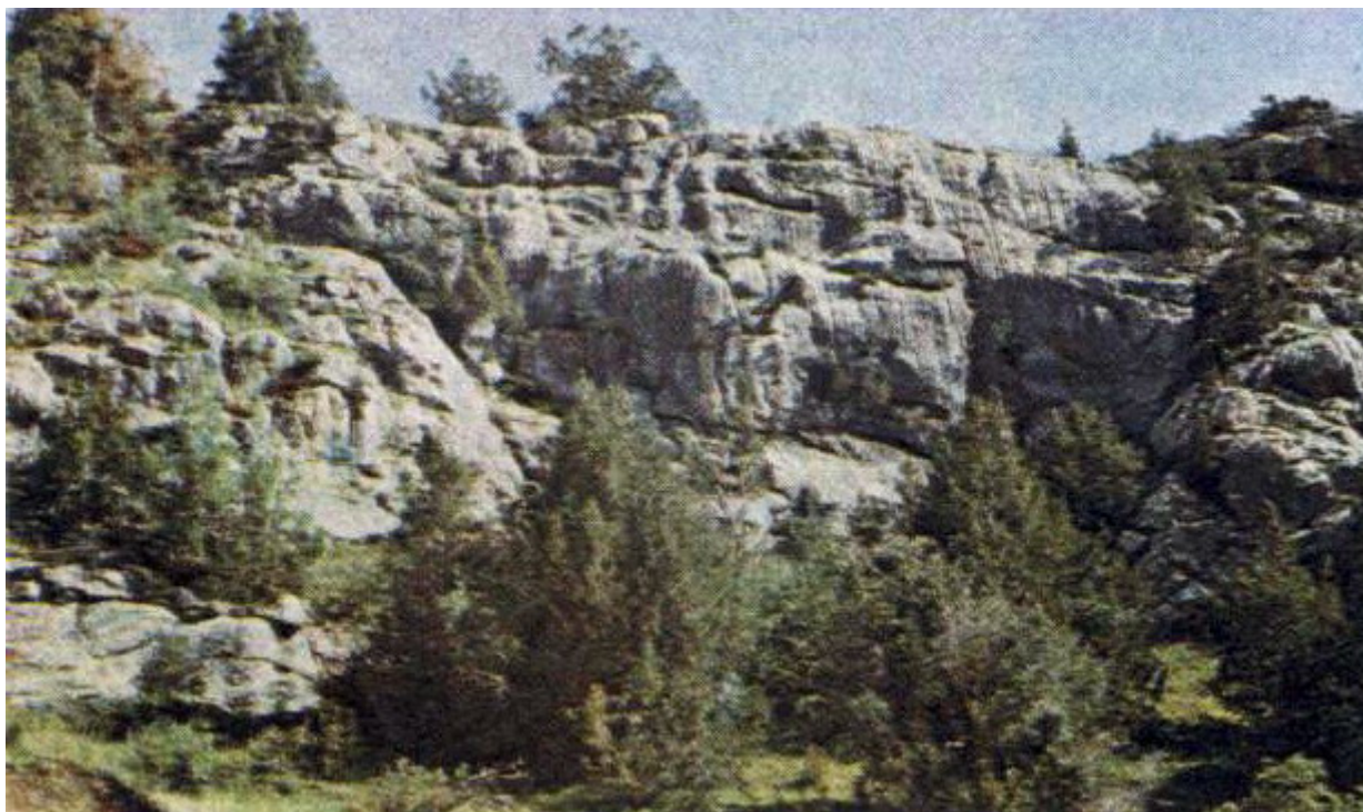
Рис. 22. Открытый карст в виде карров на карбонатной стене
