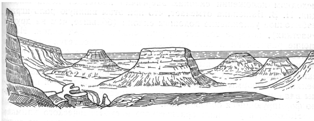
Рис.1. Структурно-денудационный рельеф Мангышлака
