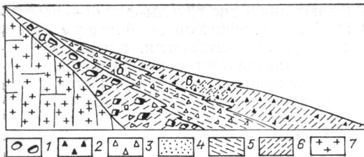
Рис. 30. Схематический разрез отложений делювиального шлейфа
