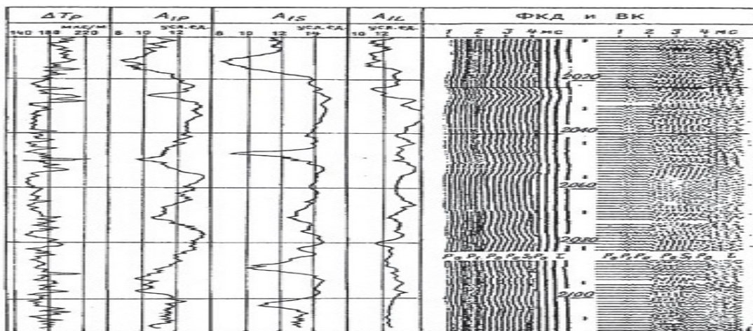
1-сурет. Карбонаттық қимадағы акустикалық каротаж нәтижелері (Ю.И.Горбачев деректері бойынша).
