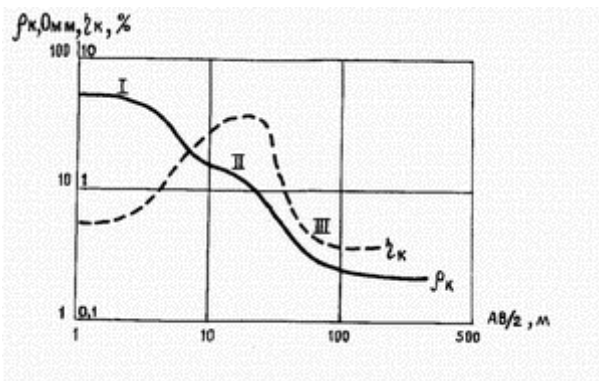
СУР. 1. ТЭЗ және ТЭЗ-ВП қисық сызық мысалы, құрғақпен негізделген(I) және сулы қабат (II) құрғақтармен, орнатылған саздар (III)
