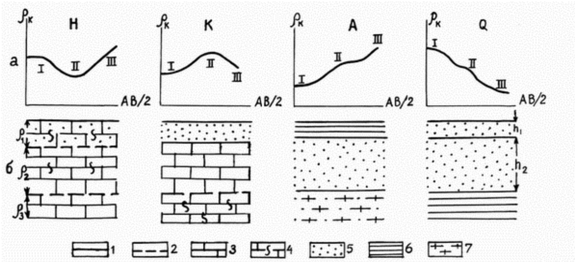
8-Сурет Қарапайым 3 қабатты ТЭЗ қисық сызығы: а – КС графигі, б – геоэлектрикалық қималар; 1 және 2 – литологиялық және гидрогеологиялық шекаралар; 3 және 4 – массивті және жарықшақты ізбестастар; 5 - құмдар; 6 - саздар; 7 – граниттер
