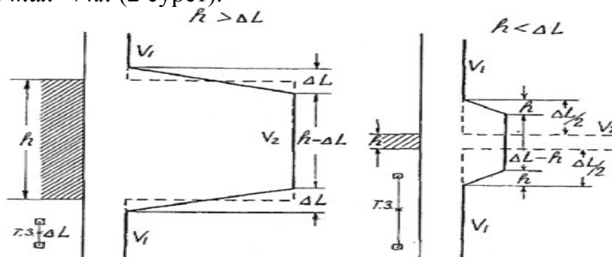
2 сурет. Толқынның жоғары таралу жылдамдығы мен сипатталатын, қалың және жұқа қабаттар үстіндегі акустикалық каротаж диаграммалары.
