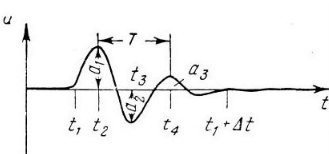
5.3-сурет Тау жынысы бөлшегінің (М) тербеліс графигі
