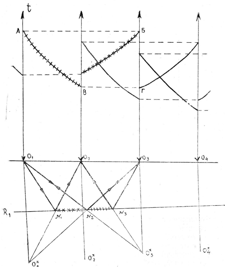
5.22-сурет Шағылған толқын әдісіндегі интервал арқылы профильдеу схемасы
