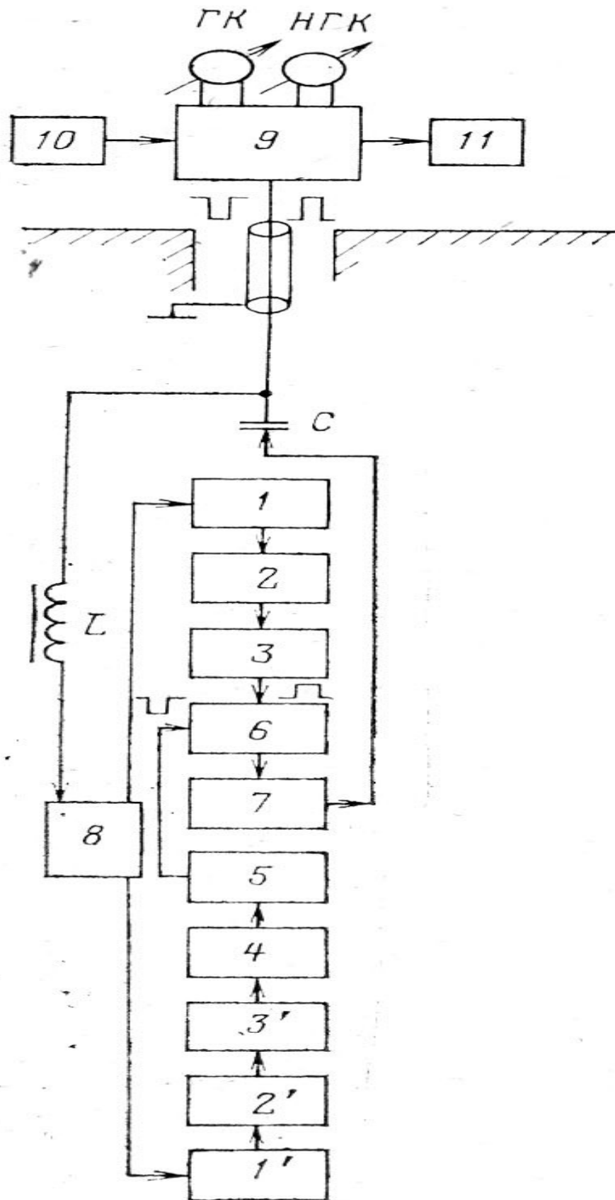
ДРСТ-аппаратурасының блок-схемасы 1 және 1 1 –ГК және НГК каналдарының санауыштары; 2 және 2 1 - күшейткіштер; 3 және 3 1 –амплитудалық дискриминаторлар; 4-триггер; 5-нормализатор; 6-сместитель; 7-соңғы (выходной)
