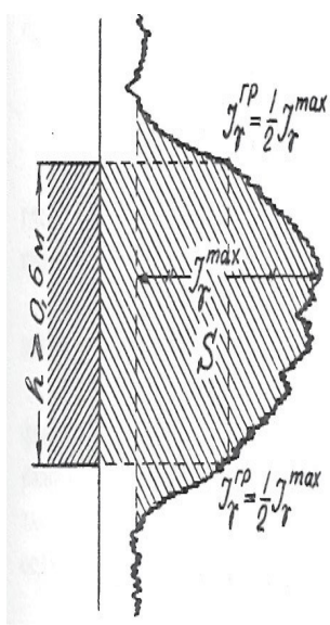
1-сурет . ГК диаграммасы бой-ынша қалың қабат жапсарлар-ын және аномалия ауданын анықтау
