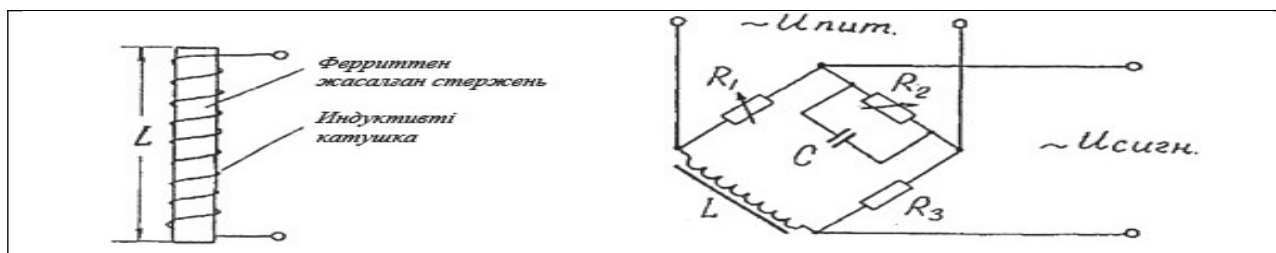
4.24 сурет КМВ аспабындағы құрылғының конструкциясы
