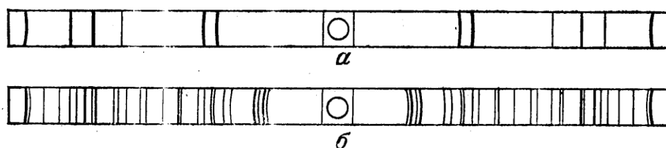
Рис. 58. Дебаеграммы: а – алмаза, б – графита.
