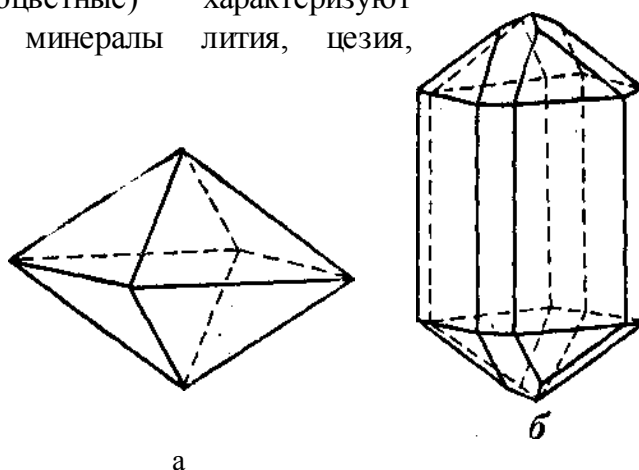
Рис. 68. Кристаллы касситерита
