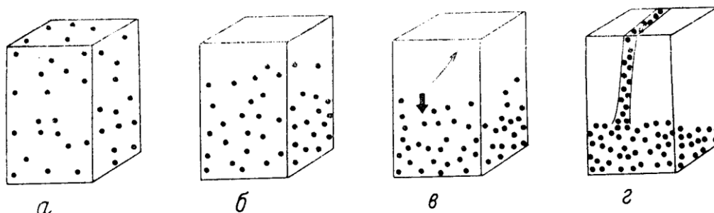
Рис.91. Схематическое изображение магматической дифференциации гранитного расплава (гранодиоритовый лампрофир) а) однородный расплав; б) осаждение тяжелых минералов; в, г) разделение тяжелой и легкой минеральных фракций. Образование кранитной и основной (габброидной) частей магм (по Г.Мабусу).
