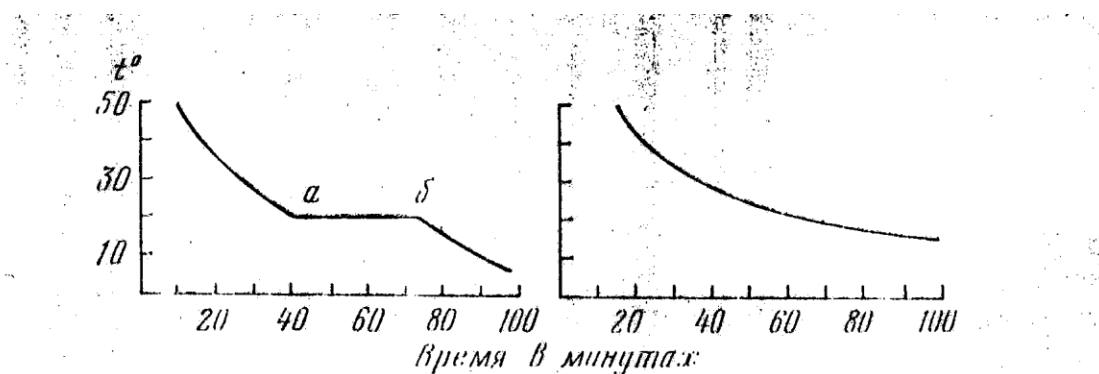
Рис. 3. Кривые охлаждения кристаллического (слева) и аморфного (справа) вещества, a и б - точки начала и конца кристаллизации
