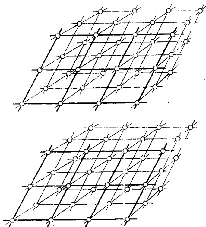
Рис. 2. Пространственная решетка
