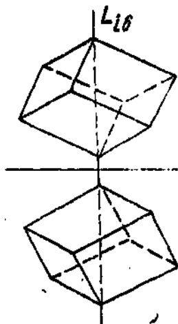
Рис. 21. Инверсионная ось шестого порядка L_{i6} или зеркально-поворотная ось третьего порядка \bar{L}_3 на ромбоэдре кальцита
