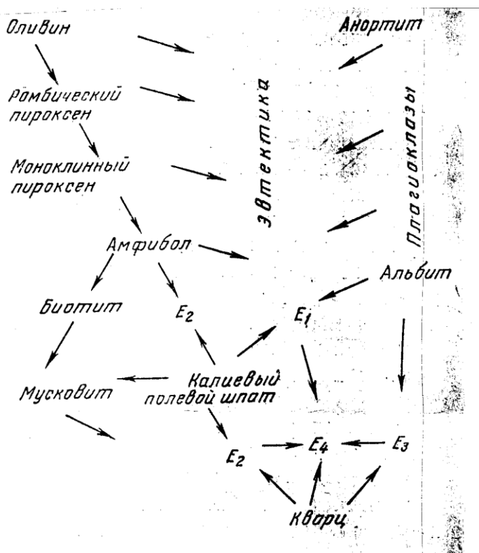
Рис. 92. А. схему последовательности кристаллизации магмы Н. Заварицкого
