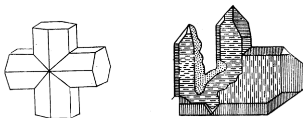
Рис. 43. Двойник прорастания у ставролита
