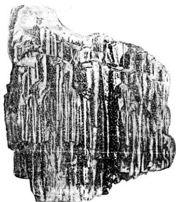
Рис. 55. Сталактит (бурый железняк)
