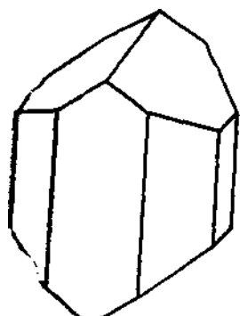
Рис. 86. Кристаллы и поперечный разрез авгита
