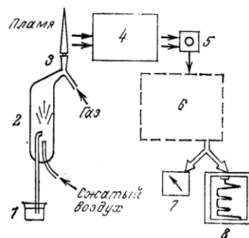
Рис. 56. Упрощенная принципиальная схема пламенной фотометрии: 1 — сосуд с анализируемым раствором; 2 — распылитель; 3 — горелка; 4 — селектор (монокроматор или светофильтры); 5 — фотоэлемент или фотоумножитель; 6 — усилитель; 7 — измерительный прибор; 8 — самописец
