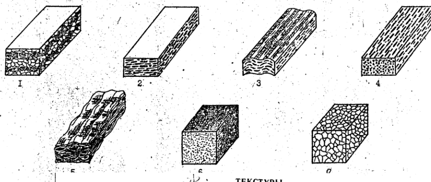
Рис.101. Макротекстуры метаморфических пород (схематические зарисовки) 1 – полосчатая; 2 – сланцеватая; 3 – пльчатая; 4 – линейная; 5 – очковая; 6 и 7 - массивная
