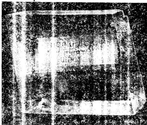
Рис. 48. Двупреломление в кристалле исландского шпата не происходит двойного светопреломления; они в оптическом отношении двuoсны .
