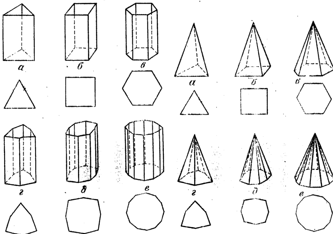
Рис. 24. Призмы средних сингоний: а — тригональная, б — тетрагональная, в — гексагональная, г — дитригональная, д — дитетрагональная, е — дигексагональная
