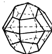
Рис. 33. Простые формы, выводящиеся из тетраэдра: \alpha – тетраэдр, \beta – тригонтритетраэдр, \theta – тетрагонтритетраэдр, \varepsilon – пентагонтритетраэдр, \delta – гексатетраэдр
