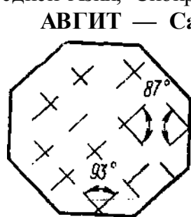
Рис. 86. Кристаллы и поперечный разрез авгита
