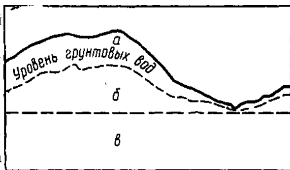
Рис. 65. Схема циркуляции подземных вод:
