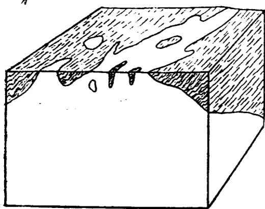
Рис.92 Батолит
