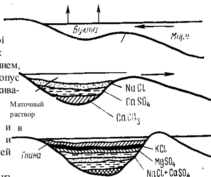
Рис. 66. Схема солеобразования по гипотезе барров:
