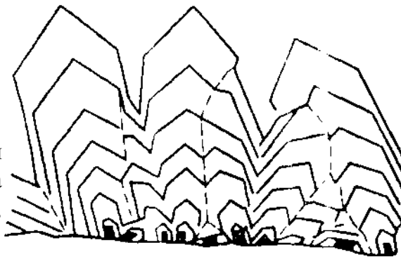
Рис. 52. Схема образования друзы горного хрусталя (по Д.П. Григорьевичу)
