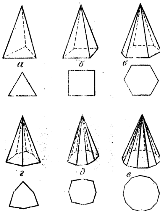
Рис. 25. Пирамиды средних сингоний: а — тригональная, б — тетрагональная в — гексагональная, г — дитригональная, д — дитетрагональная, е — дигексагональная
