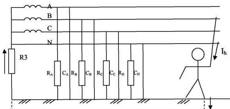
Рисунок 2– Прикосновение человека к фазному проводу
