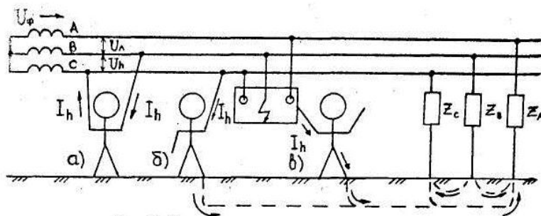
Рисунок 1 – Случайное включение человека в цепь тока:
