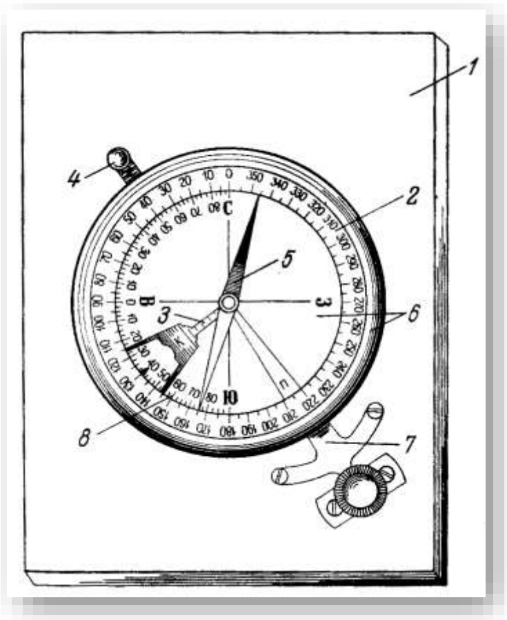
Сурет № 82 Тау құбылнамасы
