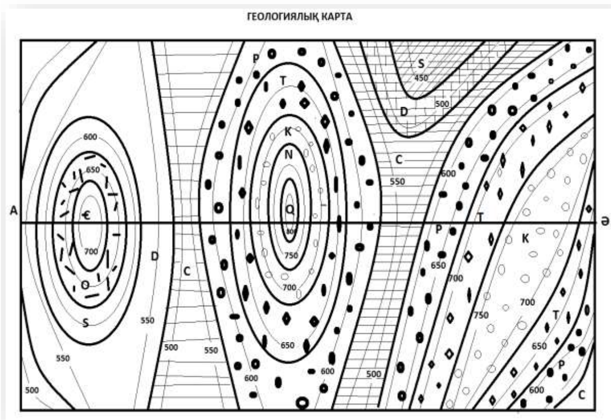
Сурет 2.1. Геологиялық карта (масштаб 1:10000)
