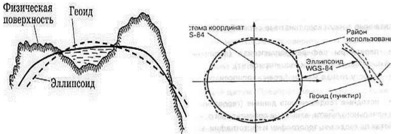
Жердің пішіні сурет № 13
