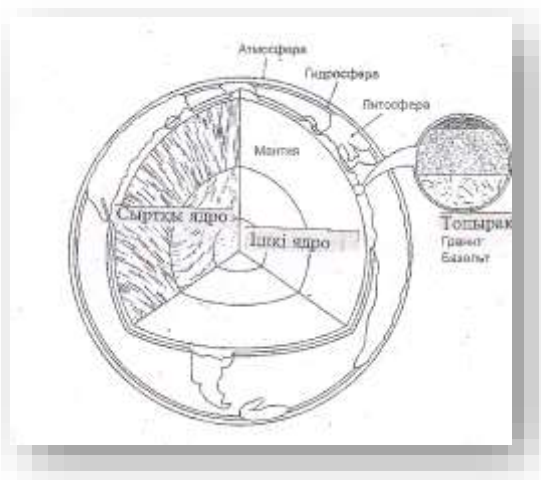
Жер қабатының сұлбасы Сурет № 17,18
