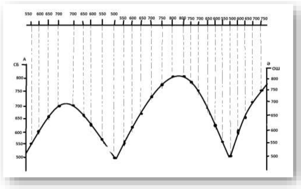
Сурет 2.2. Геологиялық қима
