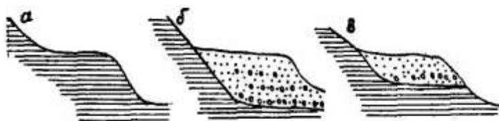
VI. 9-сурет. Өзен террасаларының түрлері: а — скульптуралық; б — аккумулятивтік; в — аралас.
