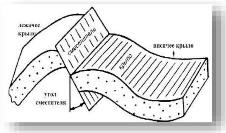
Қабаттың элементері Сурет № 89
