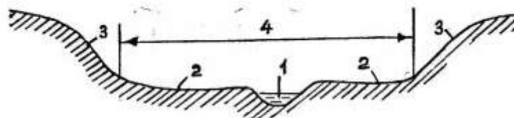
VI. 7-сурет. Өзен аңғарының элементтері: 1 — арна; 2 — жайылма; 3 — беткейлер; 4 — түп.
