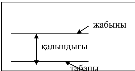
Сурет 2.3. Қабаттың элементтері
