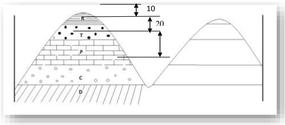
Сурет 2.4. Геологиялық қимадағы қабаттардың қалыңдығы
