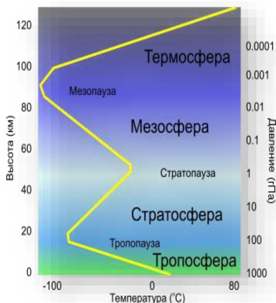
Атмосфера қабатының суреті. Сурет № 19
