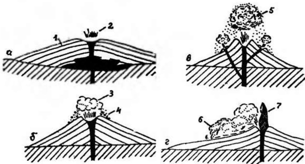
VI. 38-сурет. Вулкандық атқылаудың түрлері:
