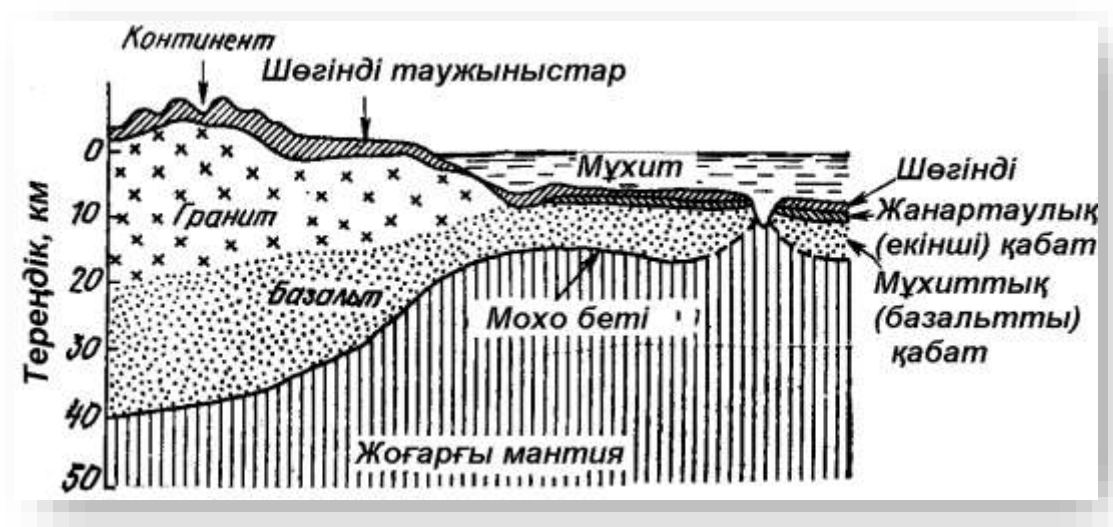
Жер қабатының сұлбасы Сурет № 17,18
