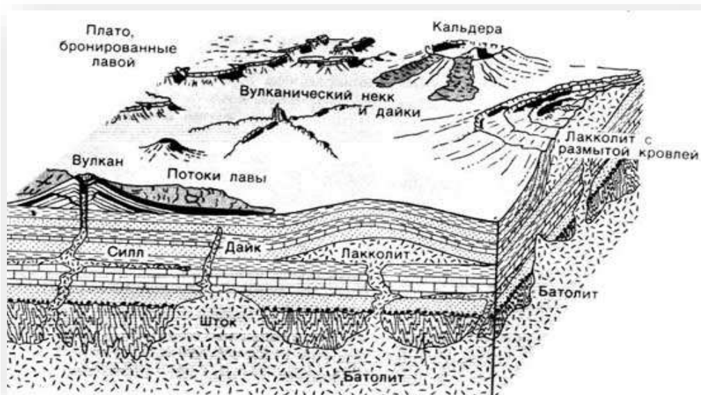
Интрузивті денелердің пішіні сурет № 64
