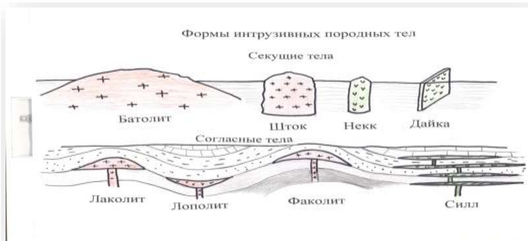
Интрузивті денелердің пішіні сурет № 64
