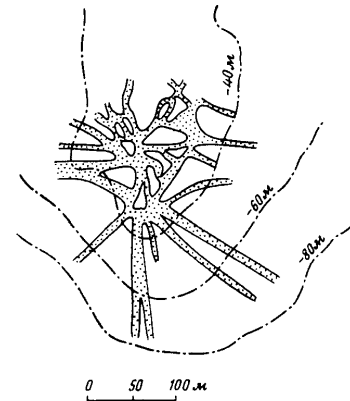
Рис. . Кластические дайки (глина) в гребце антиклинали (план) Делен, Саксония
