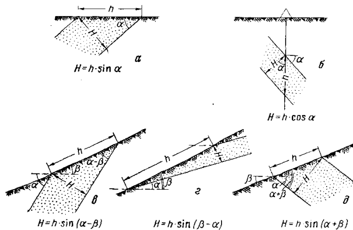
Рис. . Различные случаи определения истинной мощности наклонно залегающих слоев в сечениях, перпендикулярных простиранию слоя a - при горизонтальной поверхности рельефа, б - по керну буровой скважины, в - при наклонной поверхности рельефа (слой падает в сторону наклона поверхности рельефа, положе рельефа), г - то же, но слой падает в сторону наклона рельефа, положе рельефа; д - то же, слой падает в сторону, противоположную относительно наклона поверхности рельефа. H - истинная мощность; h - видимая мощность; \alpha - угол падения слоя; \beta - угол наклона рельефа
