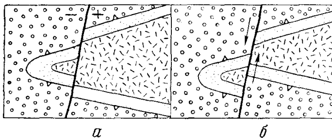
Рис. . Схемы, иллюстрирующие различие плане между сбросом (а) и сдвигом (б)
