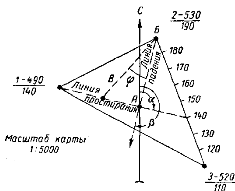
Рис. . Определение элементов залегания по трем вертикальным скважинам
