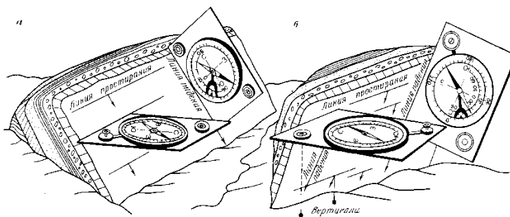
Рис. Определение элементов залегания: а - при нормальном наклонном положении слоев; б - при запрокинутом положении слоев
