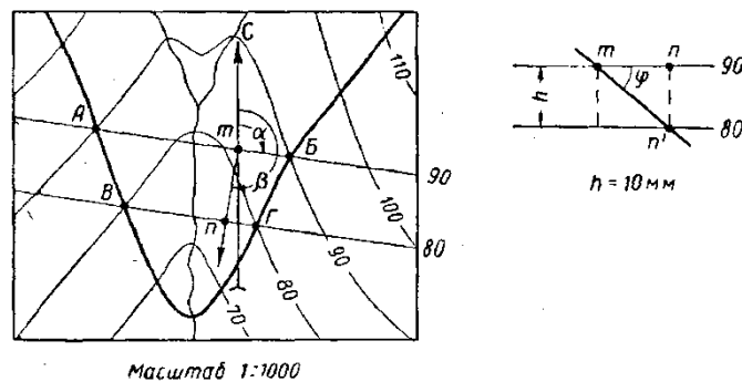
Рис. Определение элементов залегания по линии выхода пласта на поверхность с помощью заложения a - азимут линии простирания; \beta - азимут линии падения; \varphi - угол падения пласта.
