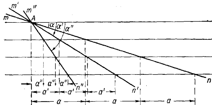
Рис. Изменение величины заложения в зависимости от угла падения слоя mn , m'n' , m''n'' - кровля или подошва пласта; \alpha , \alpha' , \alpha'' соответствующие углы падения; a , a' , a'' величина заложения
