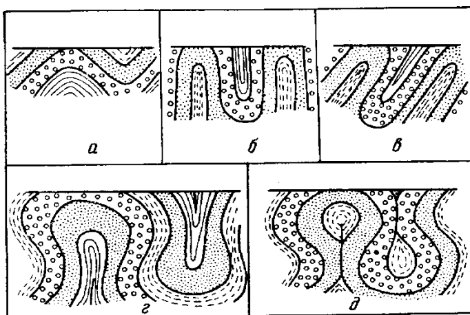
Рис. . Деление складок по соотношению между крыльями
