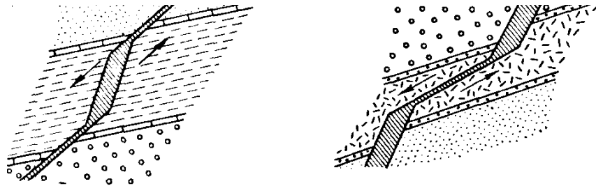
Рис. . Полости, образующиеся при перемещении крыльев сброса по искривленной поверхности смесителя
