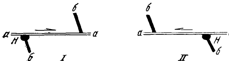
Рис. . Схема правого (I) и левого (II) сдвигов aa — поверхность сместителя; б — разорванные слои; H — положение наблюдения (плановые изображения)
