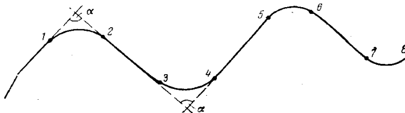
Рис. . Элементы складки
