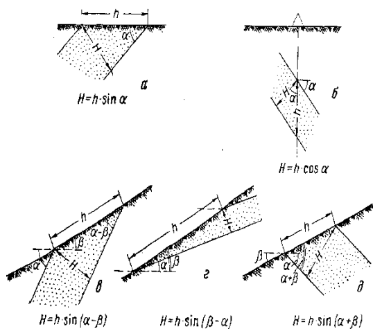
Рис.. Различные виды мощности слоя (пласта)
