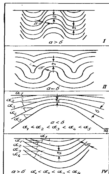
Рис. . Деление складок по соотношению мощностей на сводах и на крыльях (изображены разрезы).
