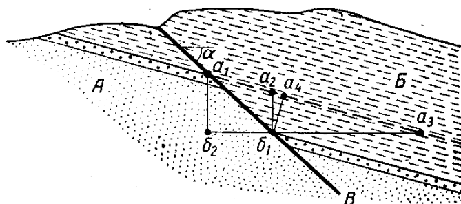
Рис. . Элементы сброса
