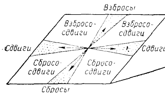
Рис. . Схема, показывающая различие в направлении смещения сбросов, сдвигов, сбросо - сдвигов и взбросо - сдвигов. Изображена поверхность сместителя. Стрелки - направление относительного смещения
