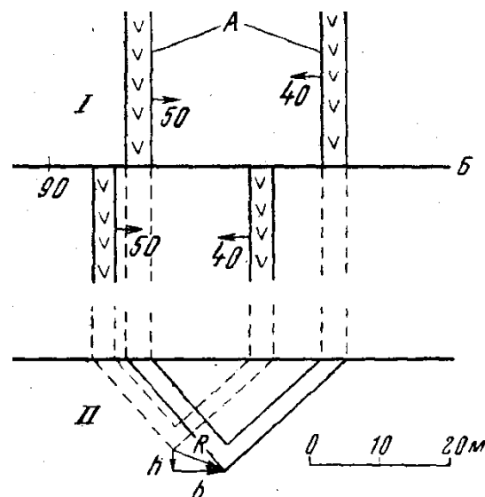
Рис. . Определение горизонтальной и вертикальной амплитуды смещения I - план двух даек лампрофиров (А), смещенных по нарушению, II - их разрез вдоль сместителя (Б)
