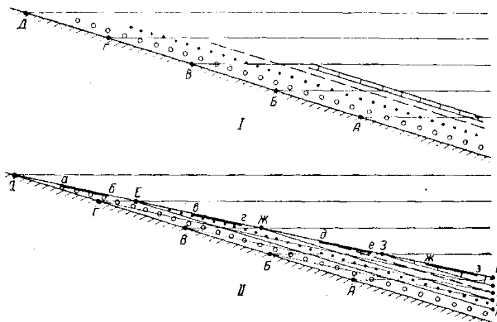
Рис. . Схема образования слоистых толщ. По Н. А. Головкинскому
