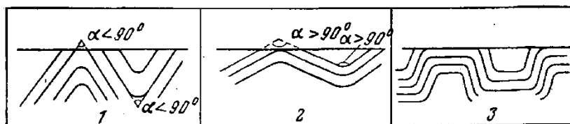
Рис. . Деление складок по форме замка (изображены разрезы) Складки: 1 — острые; 2 — пологие; 3 — коробчатые (сундучные)
