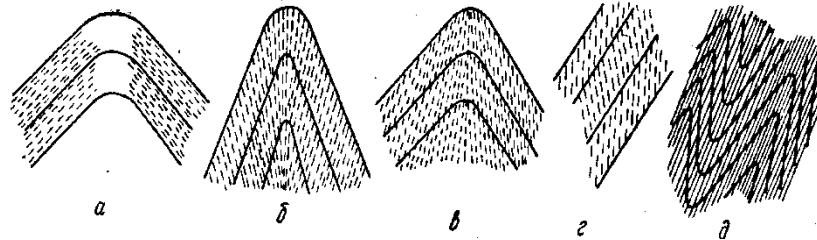
Рис. . Разновидности кливажа
