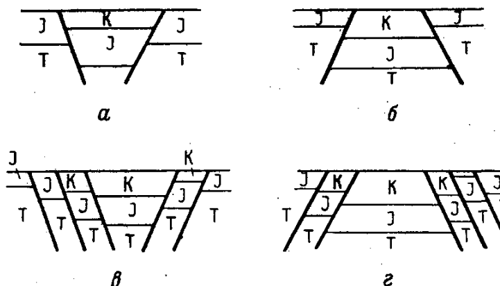
Рис. . Схемы грабенов в разрезах а - простого, образованного двумя сбросами, б - простого, образованного двумя взбросами, в - сложного, образованного сбросами, г - сложного, образованного взбросами
