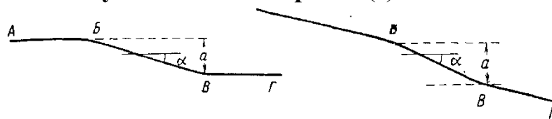
Рис. . Схема строения флексуры
