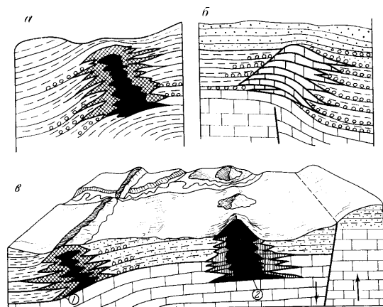
Рис. . Типы рифовых биогермных массивов и несогласные соотношения их с вмещающими породами:
