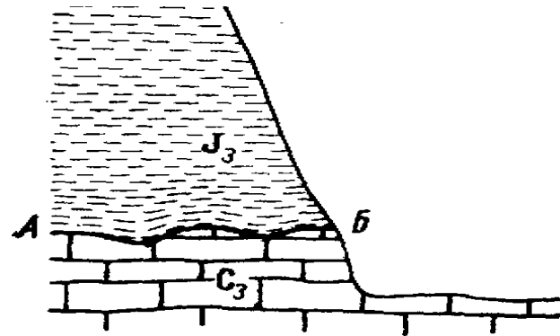
Рис. . Разрез правого берега р. Москвы (окрестности г.Москвы)
