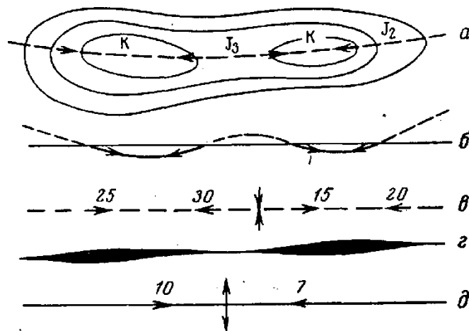
Рис. . Положение шарнира в синклиальной складке в плане (а) и в разрезе (б).
