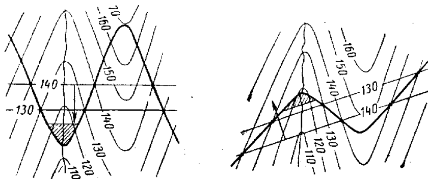
Рис. . Примеры определения направления наклона пород по пластовым треугольникам
