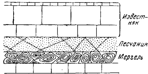
Рис. . Схема расположения первичных трещин в зависимости от состава пород.
