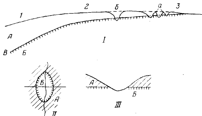
Рис. . Схема строения покрова
