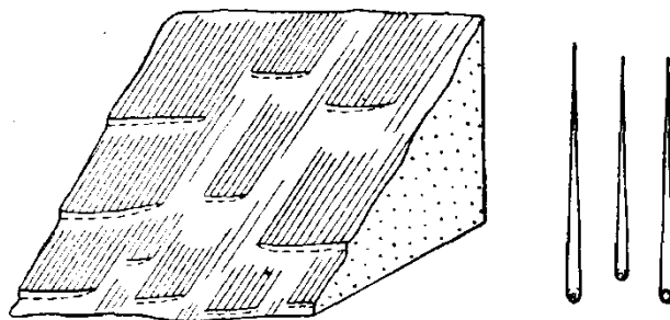
Рис. . Строение зеркала скольжения с поперечными отрывами (а) и борозд скольжения (б)
