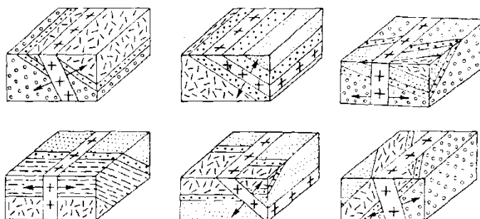
Рис. . Различные виды сочетания раздвигов и слоистости.
