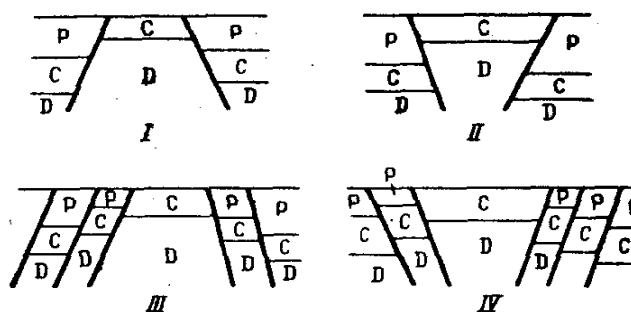
сбросами (I); простого, образованного двумя взбросами (II); сложного, образованного сбросами (III); сложного, образованного взбросами (IV)
