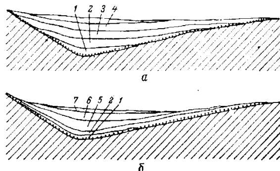
Рис. Схема строения трангрессивного (а, слои 1-4) и регрессивного (б, слои 7-5) комплексов, точечный пунктир - поверхность несогласного залегания. По М. В. Муратову
