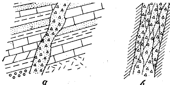
Рис. . Брекчия трения (а) и разлинзо-ванная брекчия трения (б)
