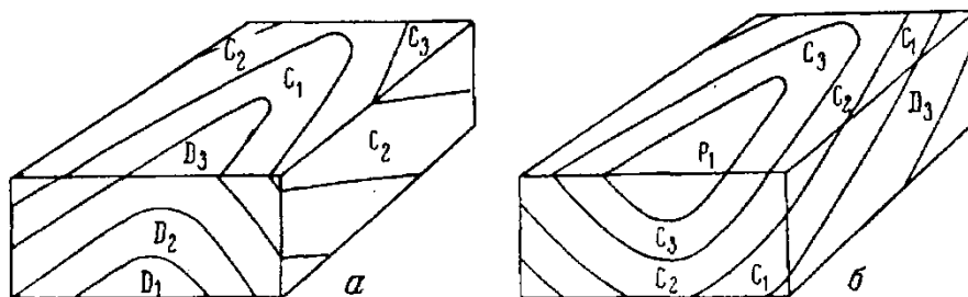
Рис. . Антиклинальная (а) и синклинальная (б) складки
